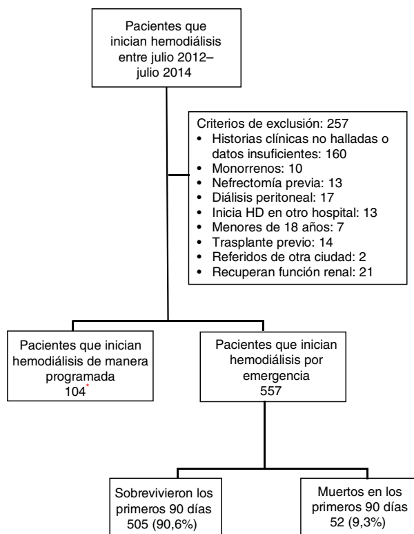
Figura 1 – Flujograma de participantes incluidos en el estudio.
