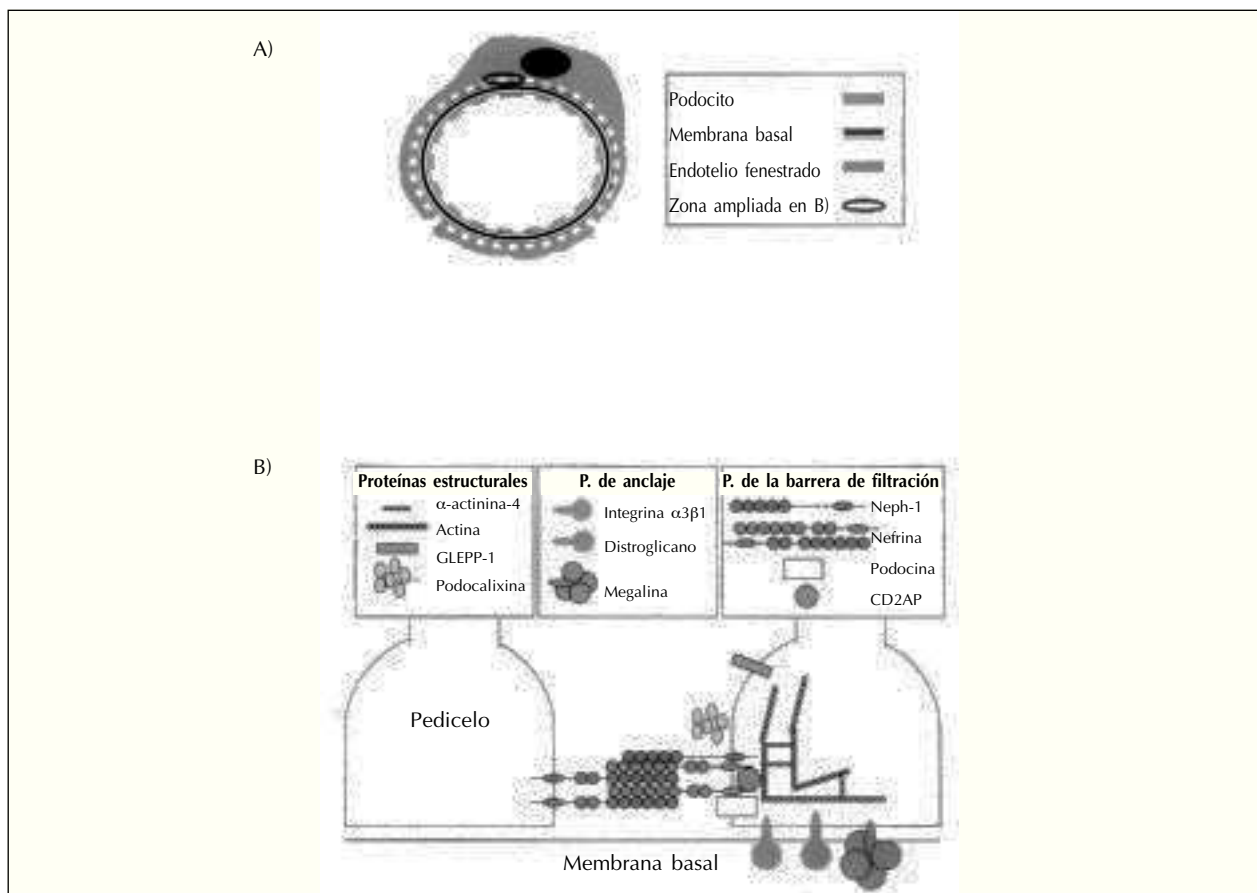
Fig. 1.—Estructura de la barrera de filtración glomerular (A) y principales proteínas conocidas responsables de la estructura y función de los podocitos, mostradas en una ampliación de los pedicelos observados en la figura A (B). Las proteínas están agrupadas según su función más probable en proteínas estructurales (mantiene la peculiar arquitectura del podocito), proteínas de anclaje a la membrana basal y proteína que forman parte de la barrera de filtración glomerular. La figura B ha sido realizada con información procedente de la referencia 6.
