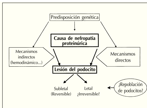
Fig. 2.—Patogenia de la lesión del podocito. Existiría una base genética que podría causar la patología glomerular o favorecer su desarrollo ante un estímulo ambiental nocivo o podría influir sobre los factores que dañan al podocito de forma directa o indirecta o en la respuesta del podocito ante la agresión. Distinguiríamos factores que dañan al podocito de forma directa, en ausencia de la contribución de la hemodinámica glomerular y de otras células glomerulares y los que lo dañan de forma indirecta a través de estos agentes. La contribución relativa de los mecanismos directos e indirectos de lesión del podocito es, en la actualidad, desconocida. La consecuencia sería una lesión letal o subletal del podocito. No existe suficiente información sobre la capacidad de regeneración del podocito.
